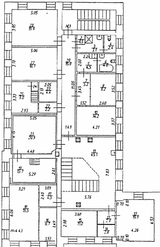
План 2 этажа
