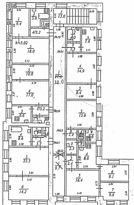
План 3 этажа
