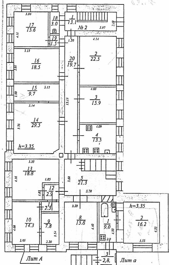
План 3 этажа
